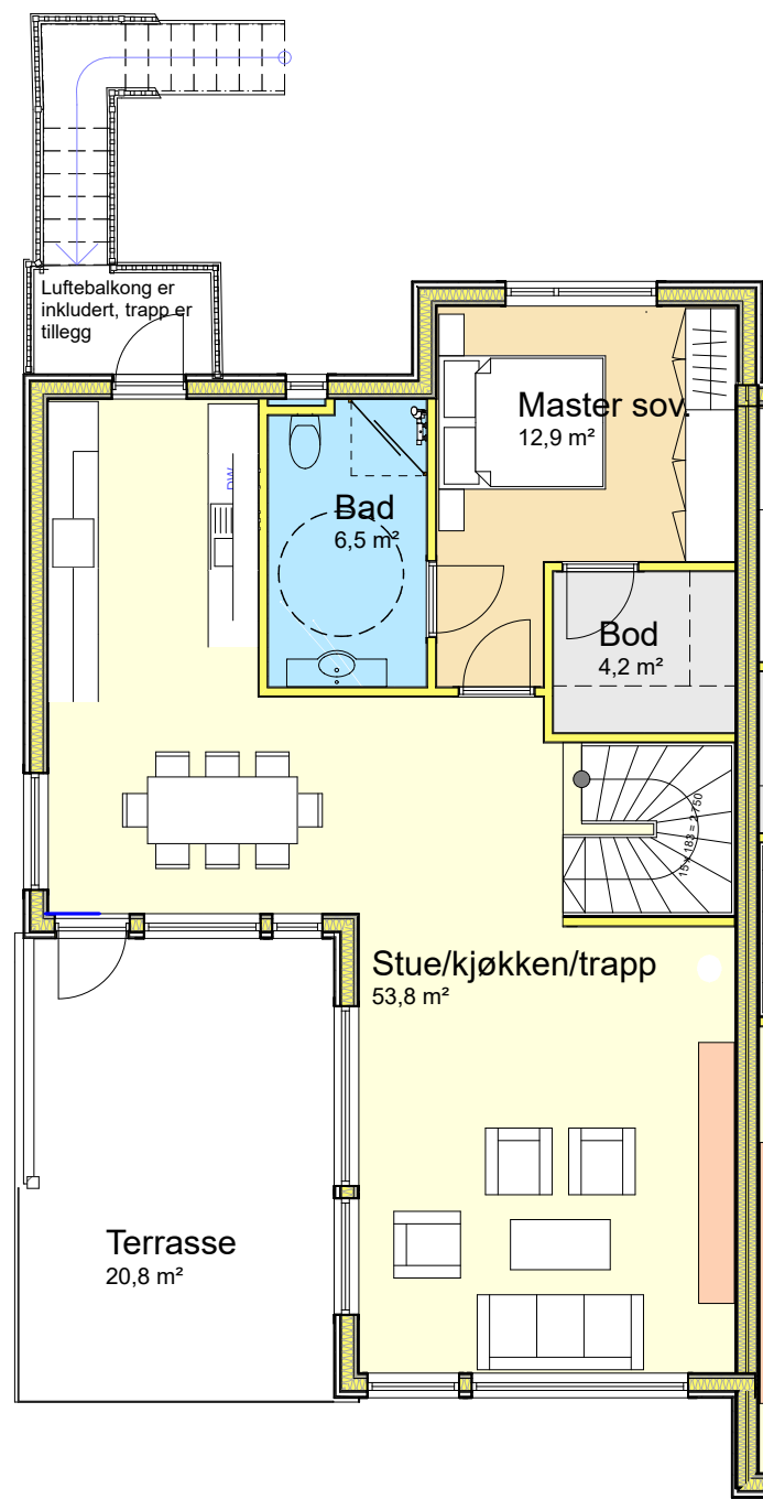
2. etasje 0 m 1 m 2 m 3 m 4 m 5 m Mål 1:100
